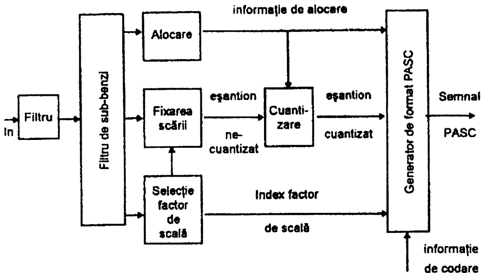
Fig.3.14 Schema bloc, de principiu, a codurii PASC.
