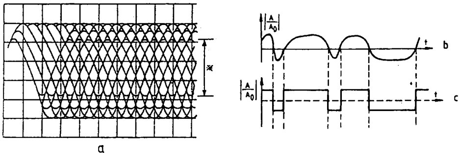
Fig.5.2 Forma semnalelor „citite” de pe banda magnetică:
