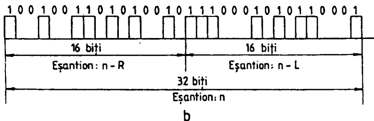
Fig.4.2 Structura semnalului inițial de AF stereo – eșantionat cu o frecvență de 48 kHz:
