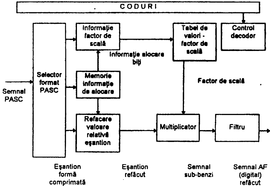
Fig.5.11 Schema bloc a decodorului PASC.
