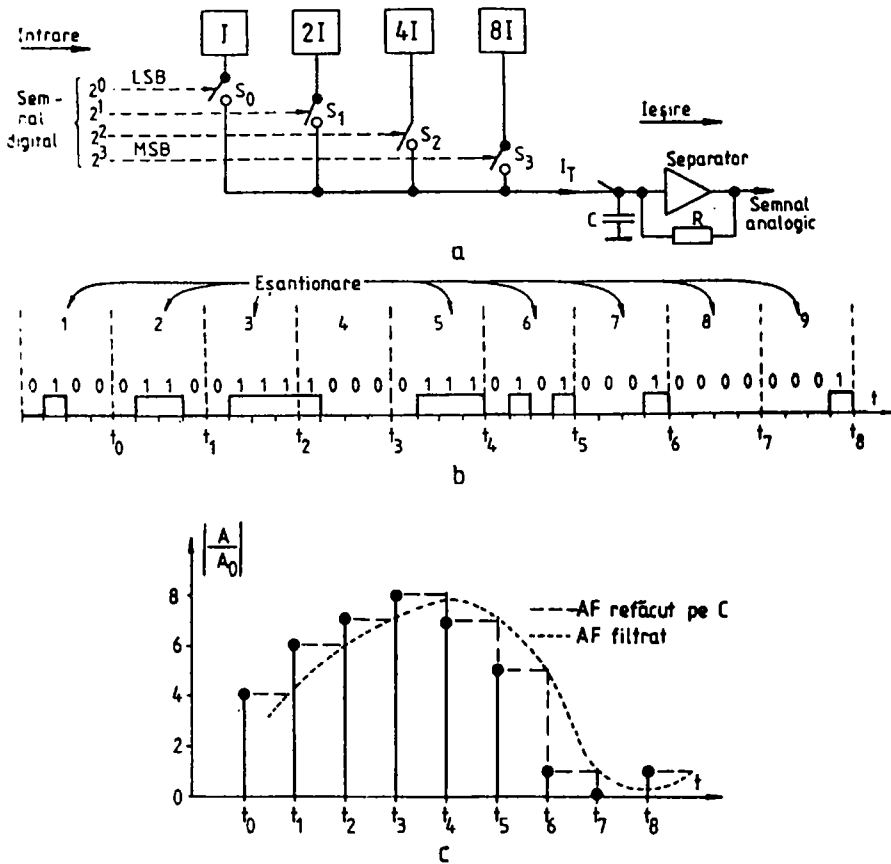
Fig.2.9 Conversia digital-analogică:
