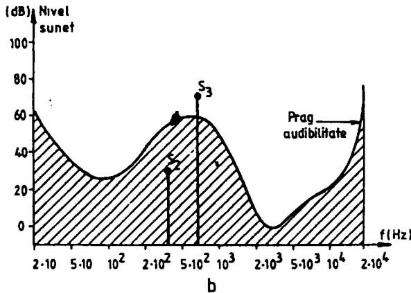
Fig.3.1 Pragul de audibilitate:
