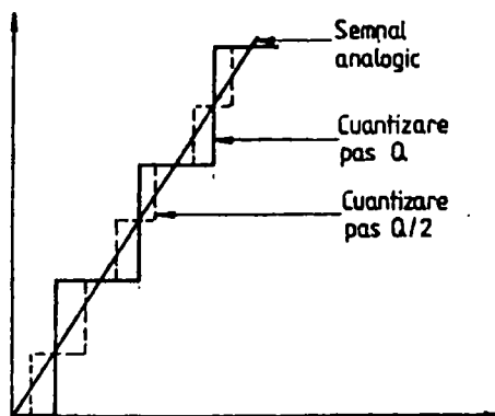
Fig.3.6 Efectul micșorării pasului de cuantizare (supraeșantionare).
