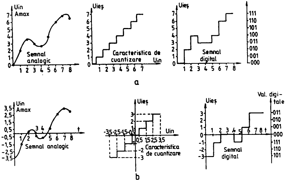
Fig.2.8 Moduri de cuantizare: a) asimetrică; b) simetrică.
