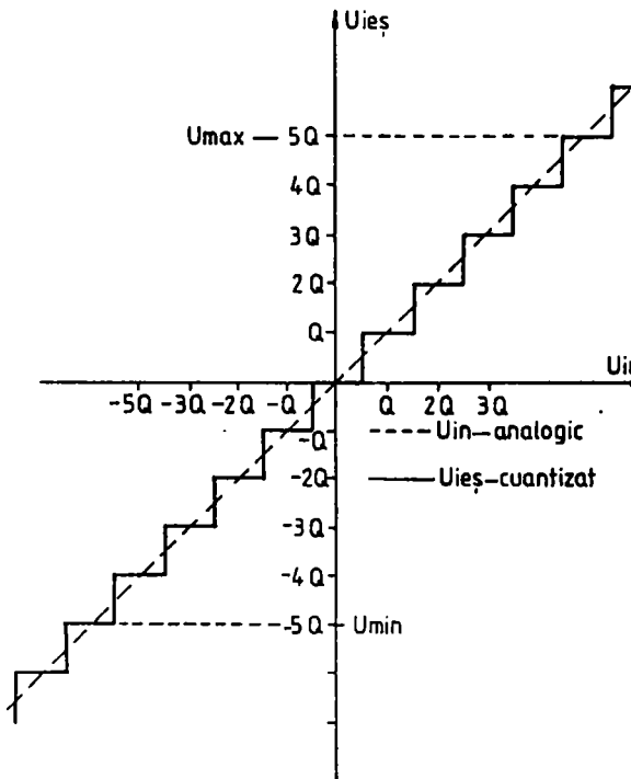
Fig.2.6 Principiul cuantizării nivelelor de semnal.
