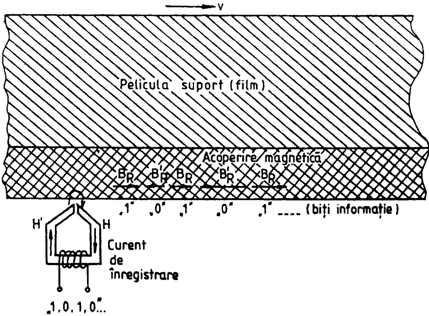
Fig.6.1 Înregistrarea-redarea semnelor digitale pe bandă magnetică.
